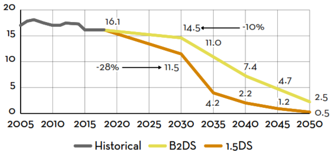
図1- アルミニウム新地金の精錬時排出量原単位の世界平均 (t CO 2 e/t Al)、2℃未満シナリオ (B2DS) および 1.5℃シナリオ (1.5DS) の場合 (AI 1.5 Degrees Scenario: A Model To Drive Emissions Reduction (AI 1.5℃シナリオ: 排出量削減推進モデル) による)
